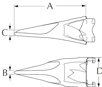
Ząb płaski komplet ESCO17
