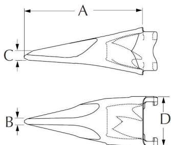
Ząb płaski komplet ESCO19
