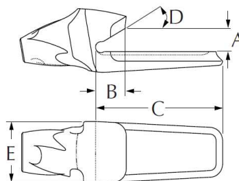
Ząb płaski ESCO19
